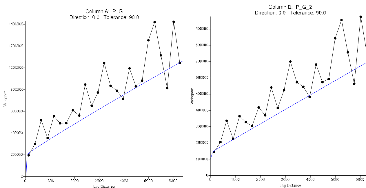
Fig. 24 – Semivariogrammi del potenziale geotermico. A destra semivariogramma per valori su 1800 h di estrazione. A sinistra semivariogramma con valori su 2400 h di estrazione.
