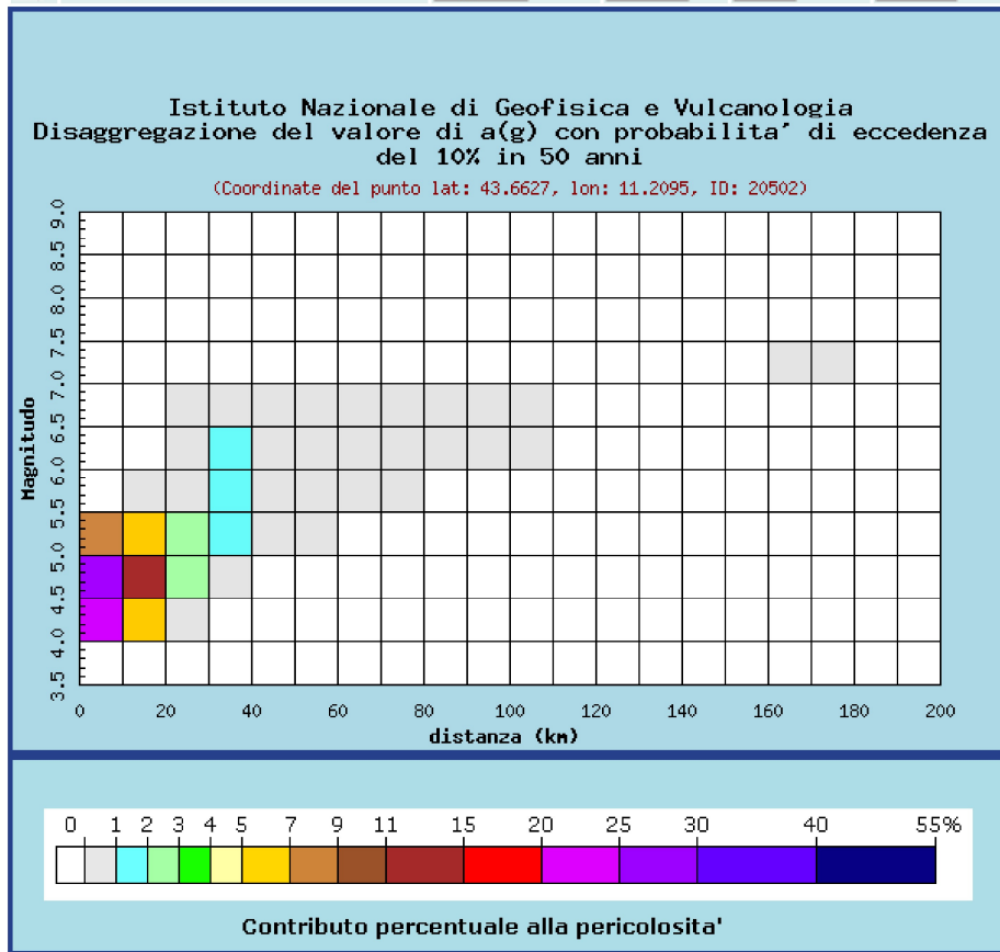
Fig. 18 – Grafico di disaggregazione del valore di ag (g) con relativa gamma di contributo percentuale alla pericolosità
